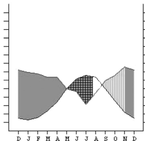
Fig. 3 - Diagramma termo-pluviometrico, utilizzo dell'acqua e caratteri bioclimatici della stazione di Firenzuola secondo l'approccio di Rivas-Martínez ( www.globalbioclimatics.org ).
