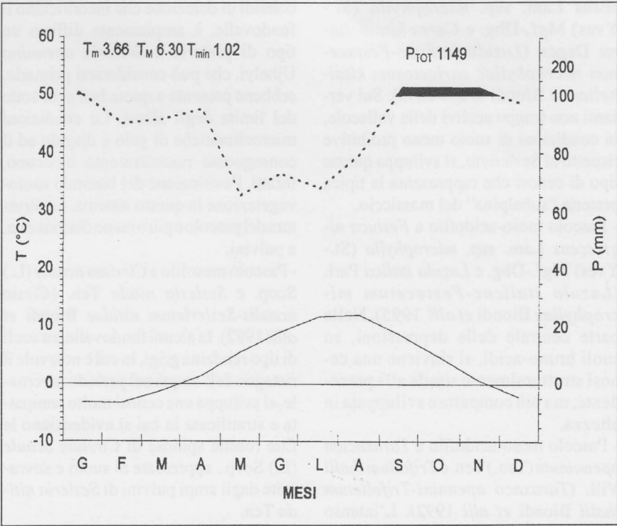
Fig. 2 — Diagramma climatico secondo Walter e Lieth (1960) modificato, media del periodo 1960-1981 ( T_m — = Temperatura media; T_M = Temperatura massima; T_{min} = Temperatura minima; P_{TOT} ..... = Precipitazione totale annua). Dati relativi alla Stazione di Campo Imperatore.
