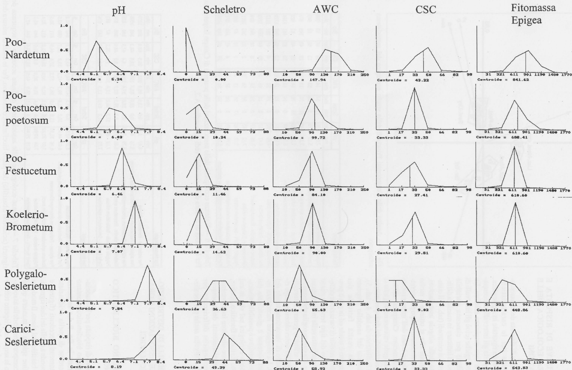
Fig. 9 — Curve di risposta per le associazioni del sottosistema montano. Per le unità di misura delle variabili vedi Appendice A.2.
