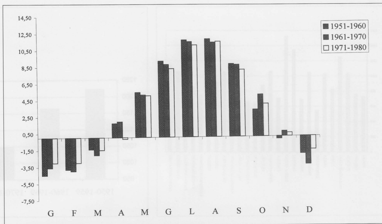
Fig. 6 — Andamento delle temperature medie mensili nella stazione di Campo Imperatore nei decenni 1951-1960; 1961-1970; 1971-1980.
