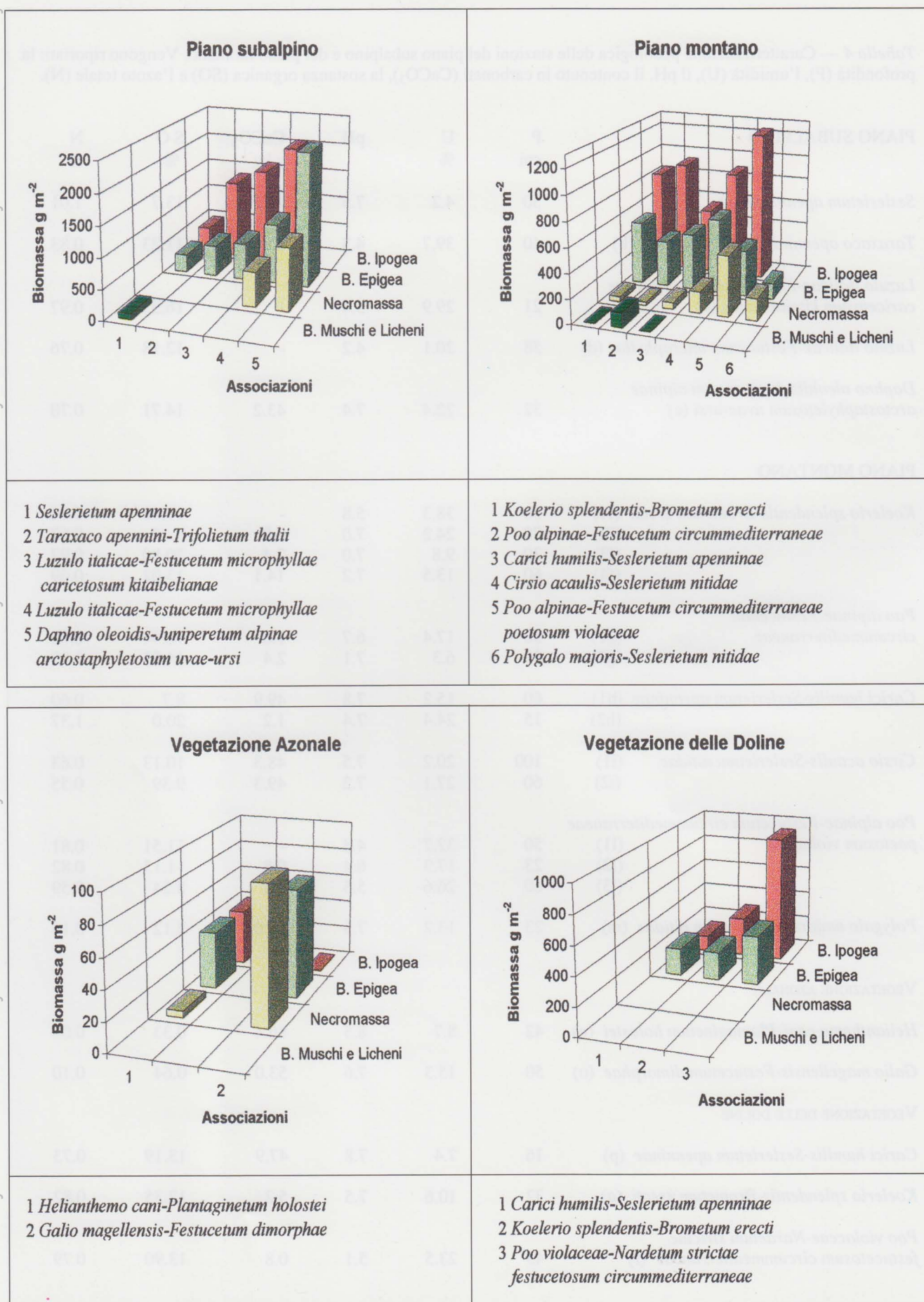
Fig. 3 — Biomassa delle associazioni esaminate.
