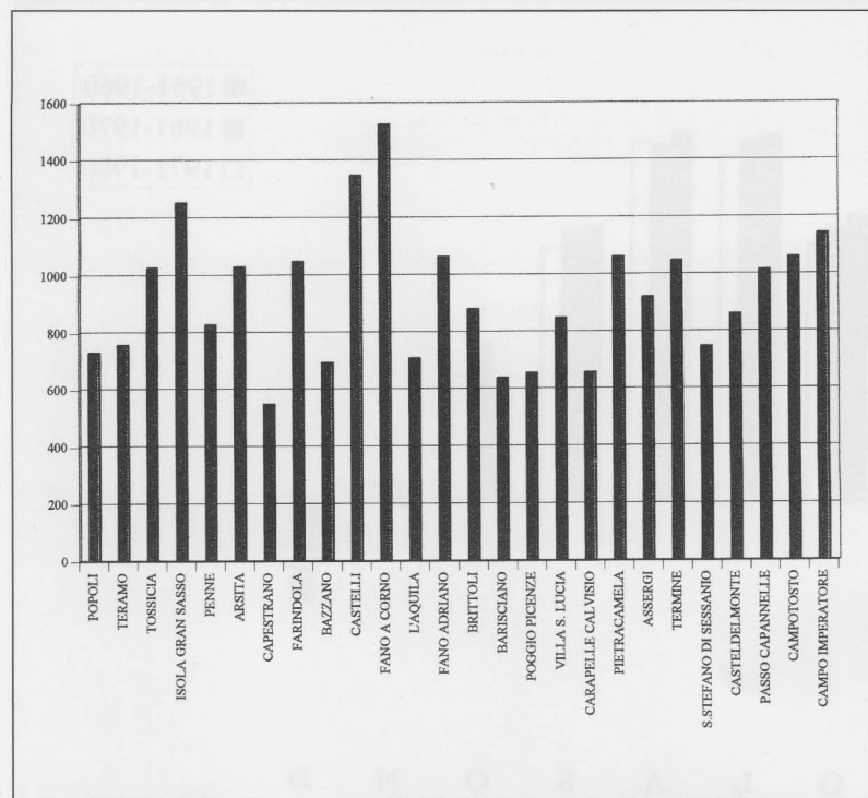
Fig. 2 — Precipitazioni medie annue (in mm) delle stazioni considerate ordinate secondo l'altitudine.
