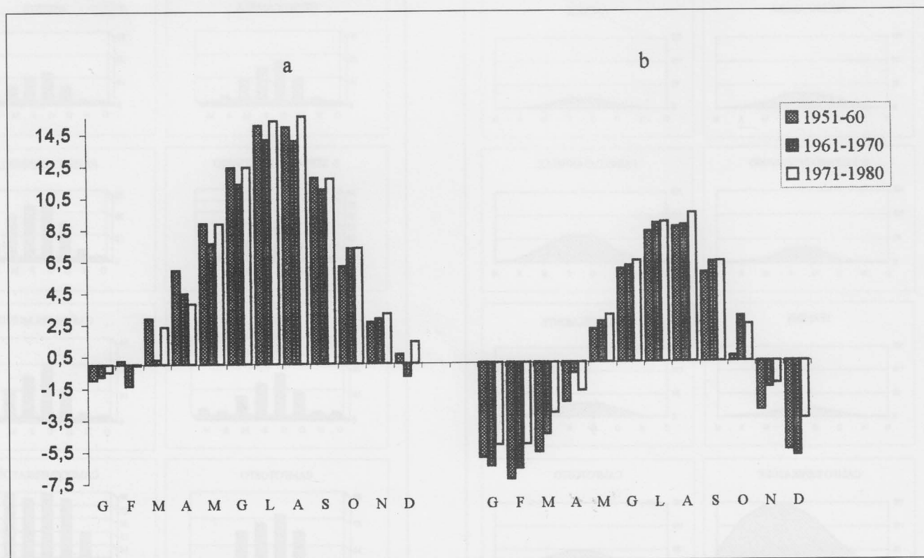
Fig. 7 — Andamento delle temperature medie mensili delle massime (a) e delle minime (b) nella stazione di Campo Imperatore nei decenni 1951-1960; 1961-1970; 1971-1980.
