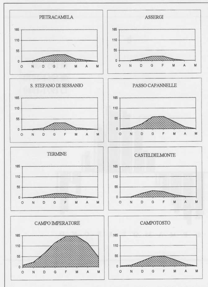
Fig. 4 — Altezza del manto nevoso (in cm) nei mesi compresi tra ottobre e maggio.
