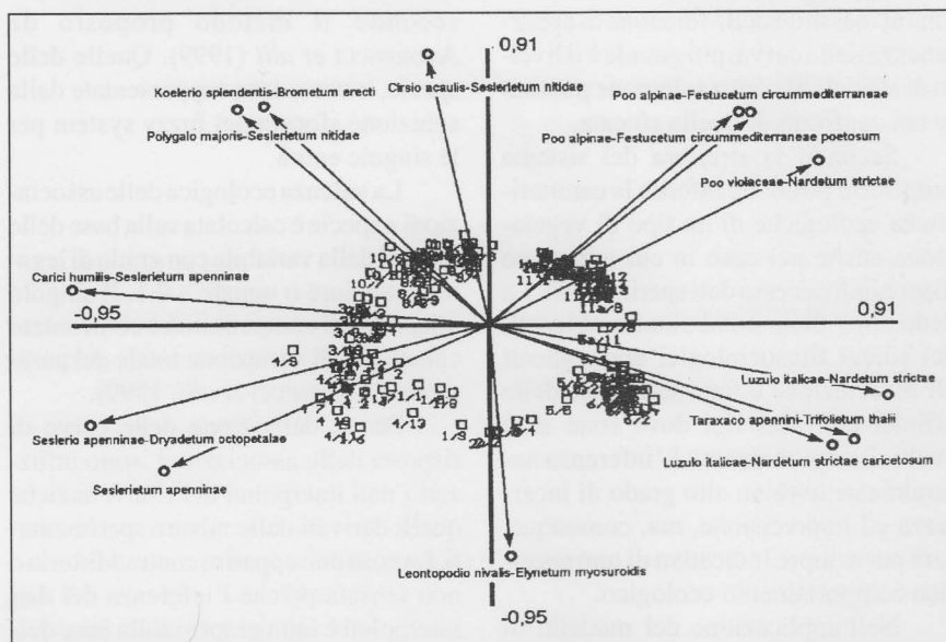
Fig. 4 — Analisi delle Componenti Principali dello spazio delle associazioni.
