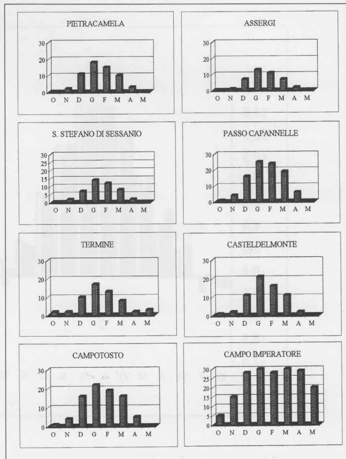
Fig. 5 — Numero dei giorni nevosi nei mesi compresi tra ottobre e maggio.
