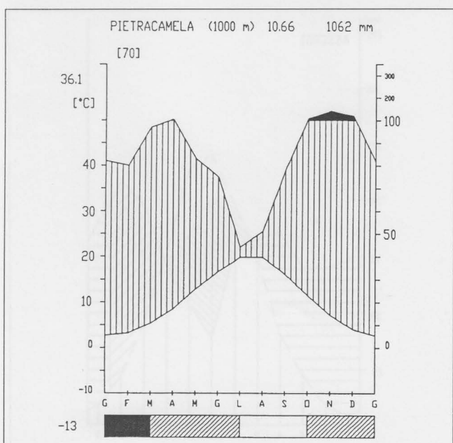
Fig. 8 — Diagrammi pluviotermici e del bilancio idrico.
