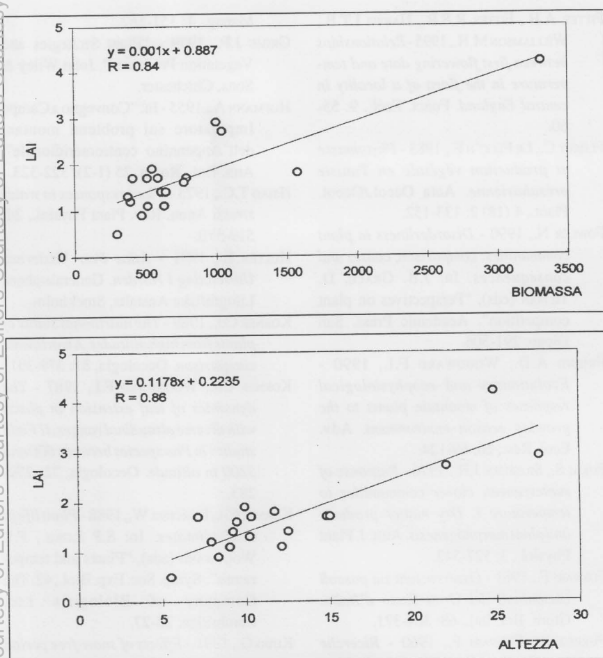
Fig. 19 — Analisi di regressione fra i valori di LAI e di biomassa e fra i valori di LAI e altezza.
