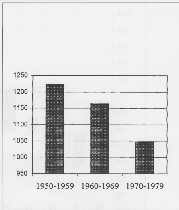
Fig. 3 — Andamento decennale delle piogge nella stazione di Campo Imperatore.
