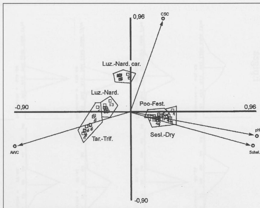
Fig. 8 — Analisi delle Componenti Principali dello spazio ecologico del sottosistema subalpino.
